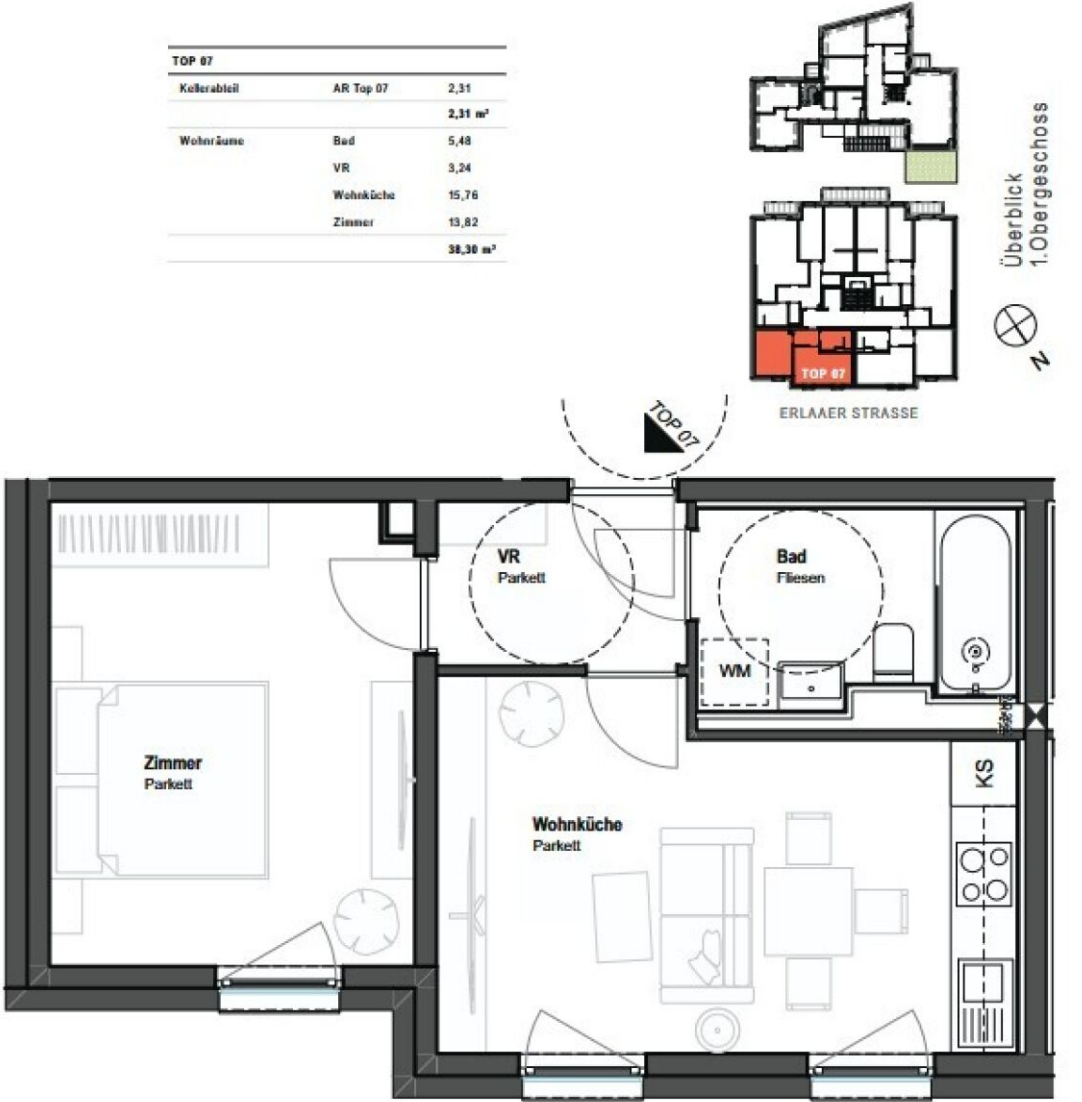
Grundriss 1:50
