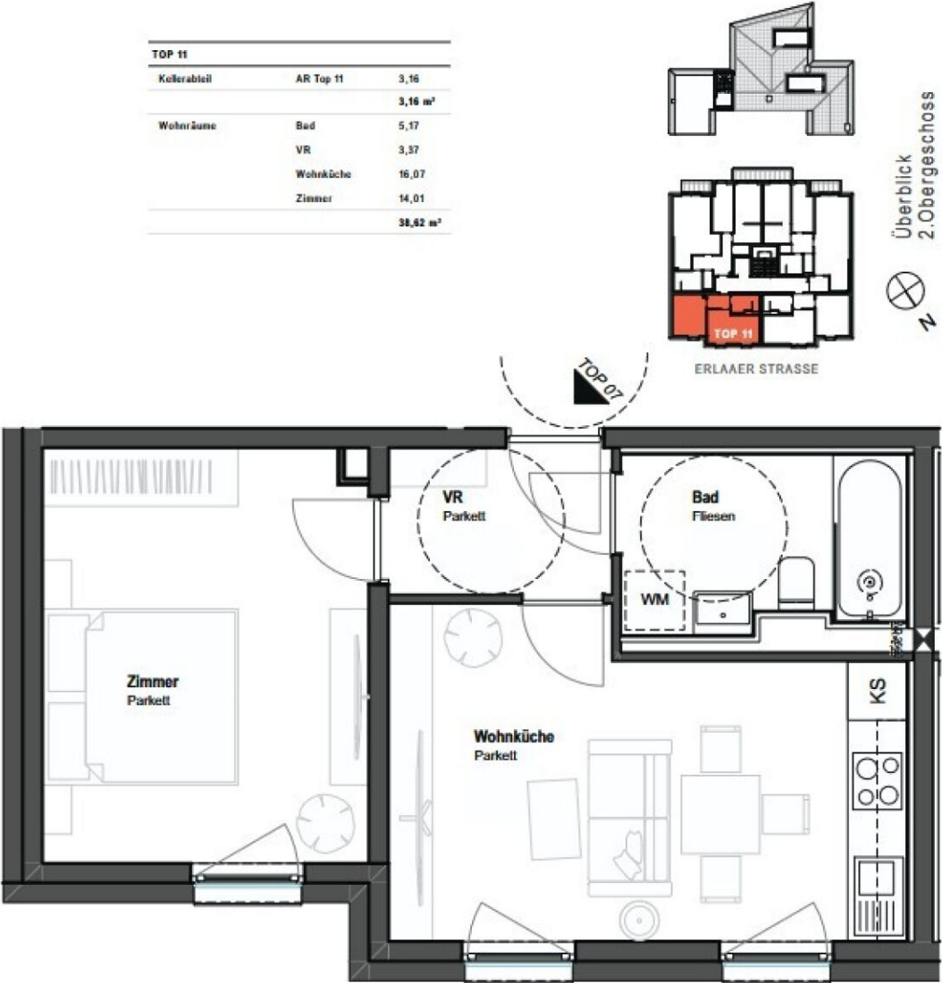
Grundriss 1:50
